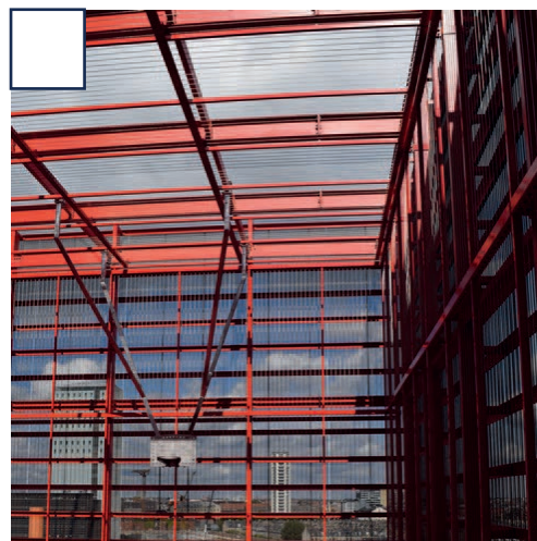
Toit composé de câbles et poutres
