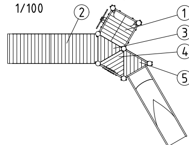
N°/orientation des planches 1/100
