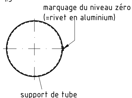
détail du marquage du niveau zéro 1:5
