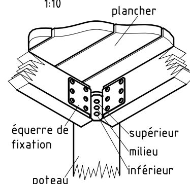
fixation des plate-formes 1:10
