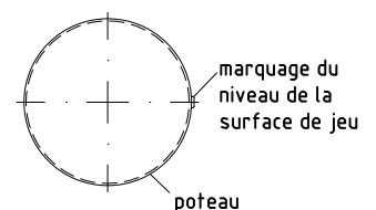
détail du marquage du poteau 1/5
