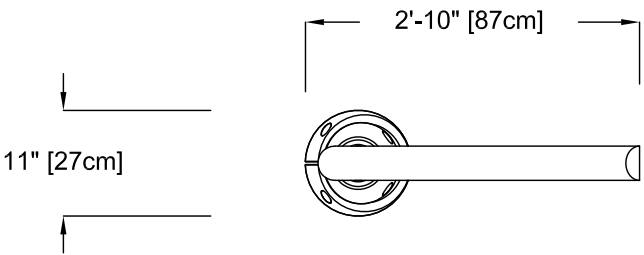
VUE D'ÉLEVATION
