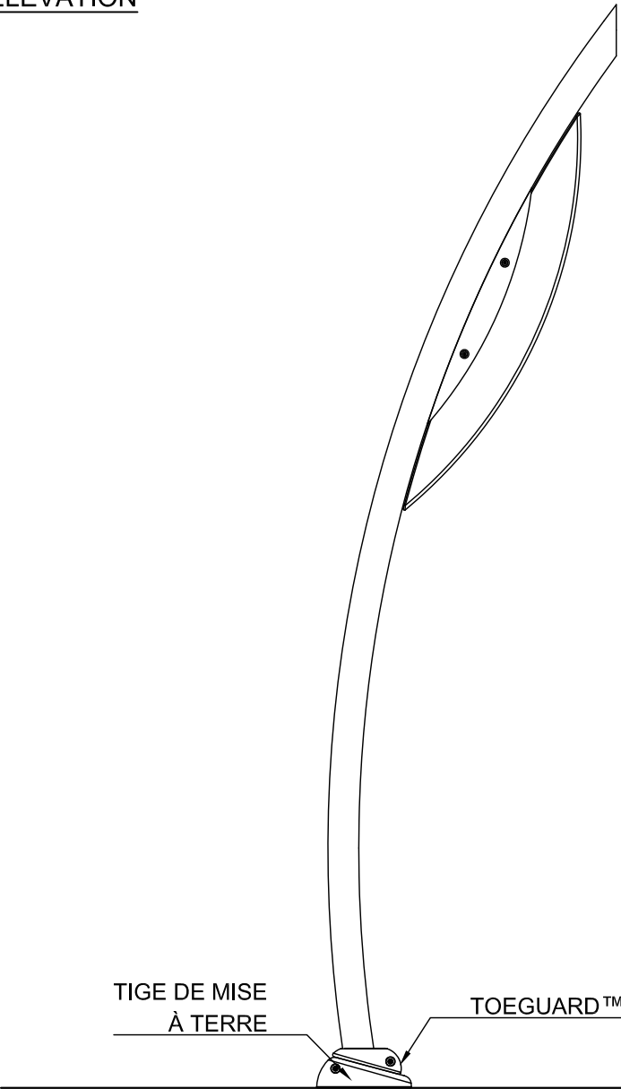
VUE D'ÉLEVATION
